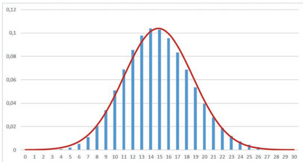
Figur 1: Binomialfordeling med n=1485 og p=0,01
